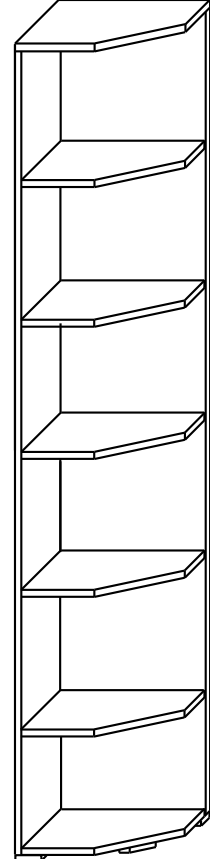
Abschlussregal inkl. 5 Einlegeböden B/H/T 40/214/40 cm
