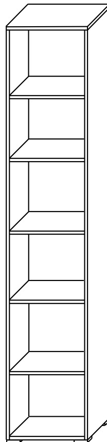
Regal inkl. 5 Einlegeböden B/H/T 42/214/40 cm
