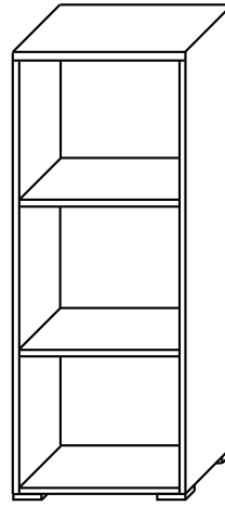
Regal inkl. 2 Einlegeböden B/H/T 42/110/40 cm
