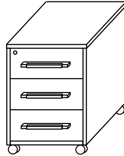
Rollcontainer auf Rollen, inkl. 3 Schubladen, obere abschließbar, B/H/T 43/59/65 cm Korpus Dekor weiß, ● Front Dekor steingrau Art.-Nr. 229662
