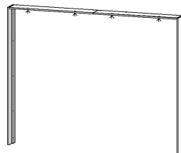
Passpartout ohne Beleuchtung Maße: B/H/T 233/214/64 cm
