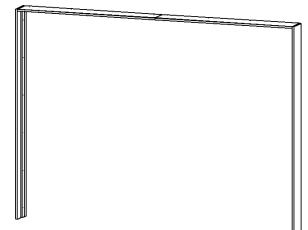
Passpartout ohne Beleuchtung Maße: B/H/T 278/214/64 cm
