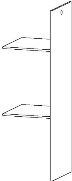
Schrankeinteilung, inkl. 2 Stoffkisten mit 2 Fachböden, für Elementbreite 90 cm Maße B/H/T: 45/147/48 cm Art.-Nr. 564066
