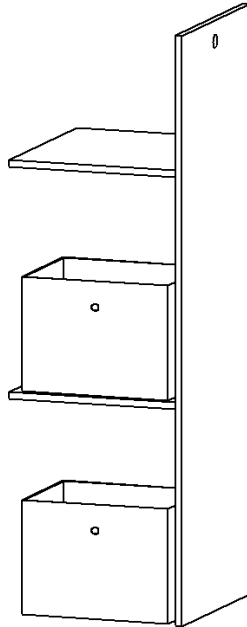
Schrankeinteilung, inkl. 2 Stoffkisten mit 2 Fachböden, für Elementbreite 90 cm Maße B/H/T: 45/147/48 cm Art.-Nr. 564066
