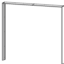
Passpartout ohne Beleuchtung Maße: B/H/T 278/233/64 cm
