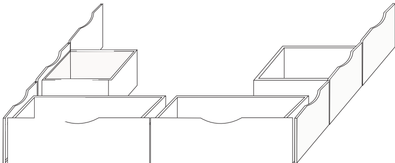
Bettkasten-Set, mit 4 Schubladen Maß: B/H/T 180/28/203 cm
