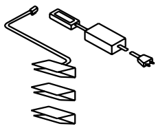
LED-Graskantenbeleuchtung, mit 20 weißen Doppelpunkt LED's, Anbauwand-Komplett-Set, inkl. Trafo und Zuleitung, Art.-Nr. 327106
