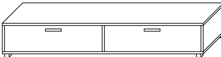
Unterteil, Korpus Nachbildung Kernnussbaum, mit zwei Schubladen cremeweiß lackiert, Maße: B/H/T 177/27/50 cm Art.-Nr. 280418
