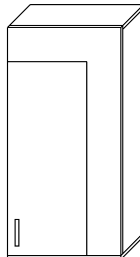
Hängeelement, Korpus Nachbildung Kernnussbaum, mit einer Tür cremeweiß lackiert, Tür links angeschlagen, Maße: B/H/T 60/122/37 cm Art.-Nr. 280422
