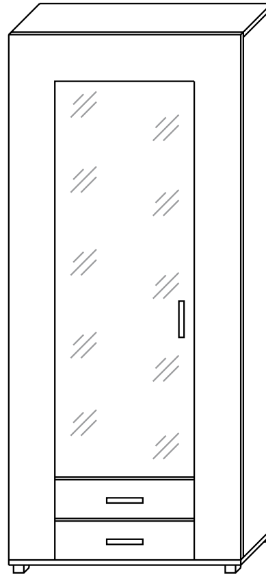
Vitrine, Korpus Nachbildung Kernnussbaum, mit einer Klarglastür und zwei cremeweiß lackierten Schubladen, Tür links angeschlagen, Maße: B/H/T 90/205/37 cm Art.-Nr. 280417
