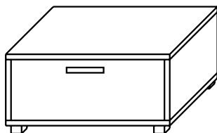
Unterteil, Korpus Nachbildung Kernnussbaum, mit einer Schublade cremefarbig lackiert, Maße: B/H/T 60/27/50 cm Art.-Nr. 280420
