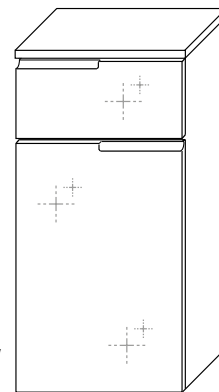
Unterschrank, Korpus weiß, Front Hochglanz Lack weiß, eine Tür, eine Schublade, Maße: B/H/T 40/86/32 cm Art.-Nr. 651204
