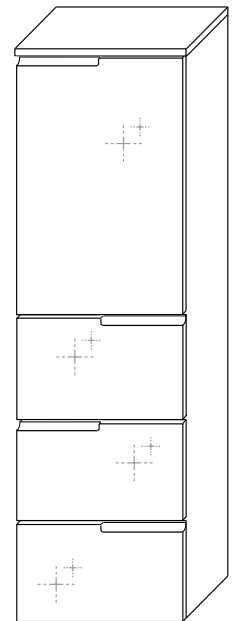
Hochkommode, Korpus weiß, Front Hochglanz Lack weiß, 3 Schubladen und eine Tür, Maße: B/H/T 40/134/32 cm Art.-Nr. 651222
