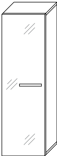
Hängeelement, Korpus schwarz, mit einer Schwarzglastür Maße: B/H/T 39/128/30 cm Art.-Nr. 142184
