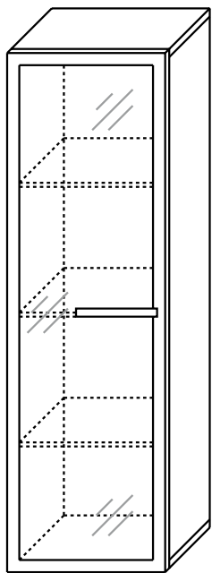
Hängeelement, Korpus schwarz, mit einer Tür in Parasolglas grau Maße: B/H/T 39/128/30 cm Art.-Nr. 142186
